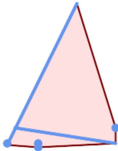
多线串和多点的凸包
