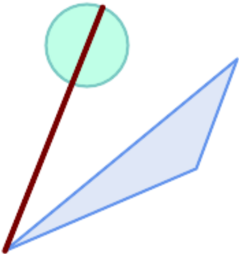
一个多边形之最长的线
