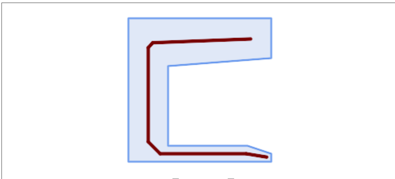
多边形及其近似中线
